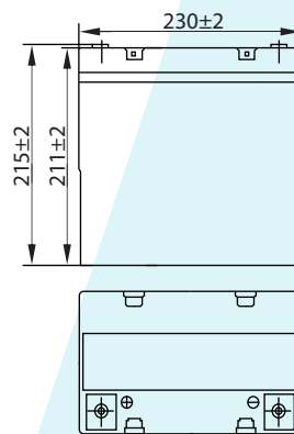
РАЗМЕРЫ
