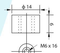
КЛЕММ Т16
