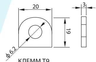
КЛЕММ Т9
