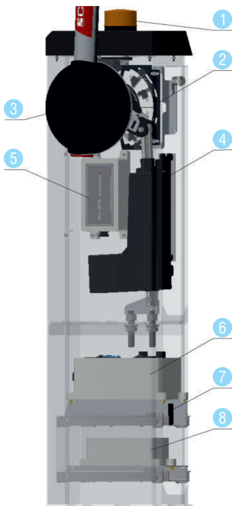
Рисунок 6.1 Внешний вид и состав шлагбаума
