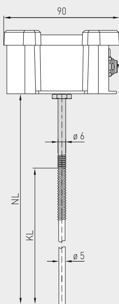
MWTM-EtherCAT P
