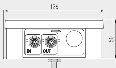
Габаритный чертеж
