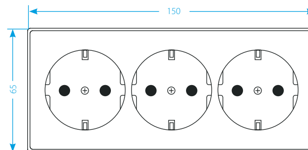
Тройная розетка IP20
