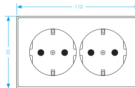
Двойная розетка IP20
