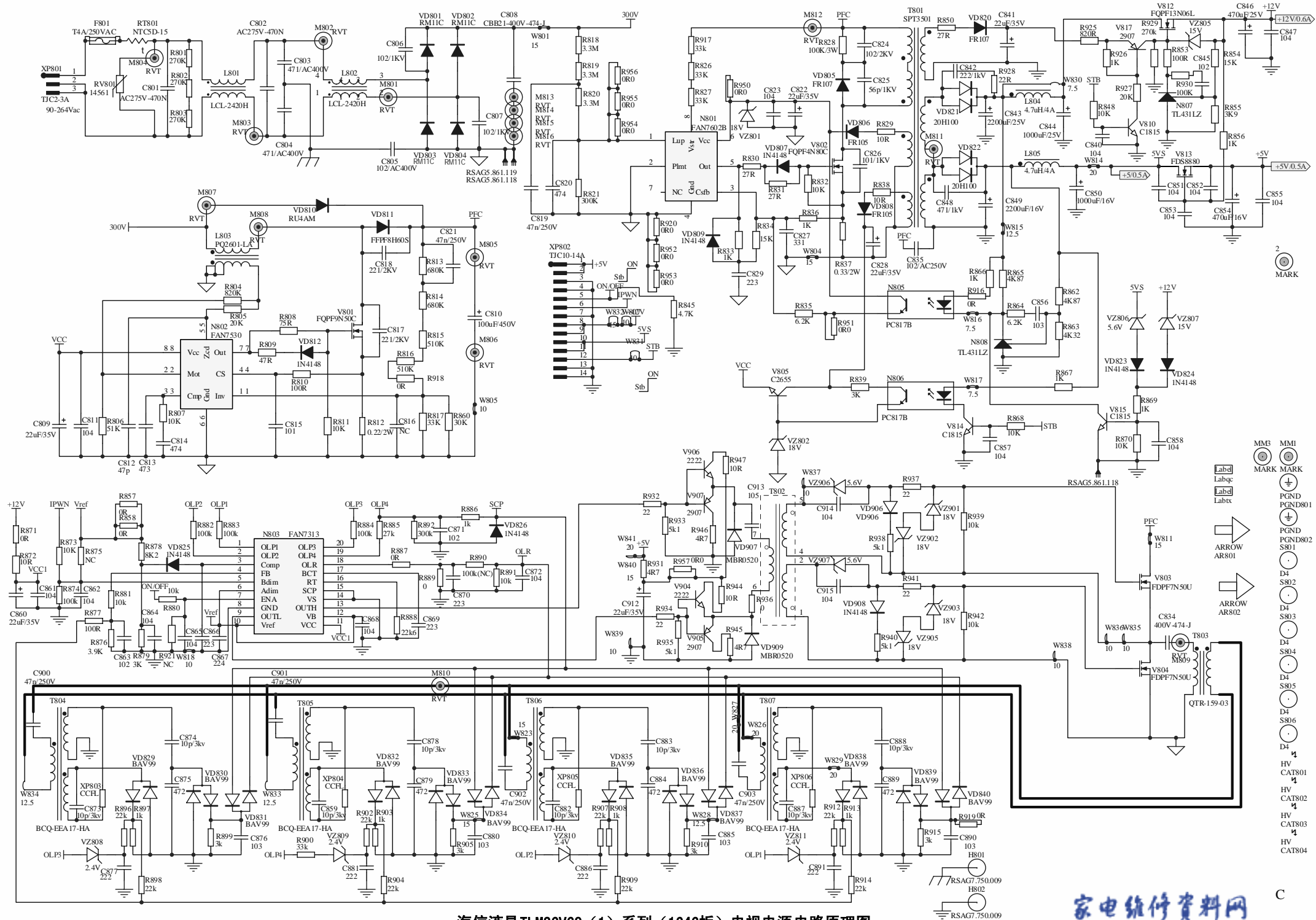
海信液晶TLM26V68 (1) 系列 (1646板) 电视电源电路原理图
