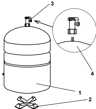
Рисунок 6. Накопительный бак
