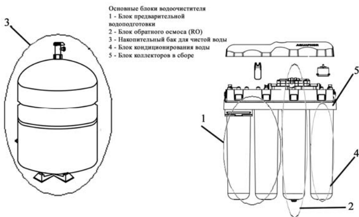
Рисунок 1. Устройство водоочистителя
