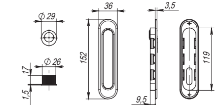
SH010-AB-7 Бронза
