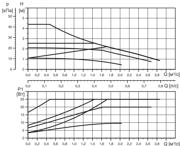
16-сур. ALPHA1 L сериясындағы сорғылардың шығынды-арынды сипаттамасы
