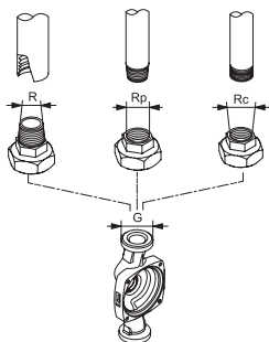
Рис. 21 Резьба G и резьба R
