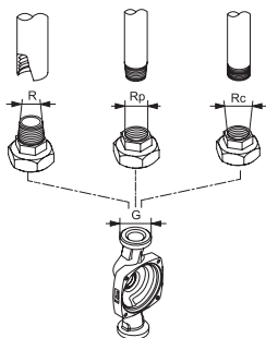
21-сур. G резьбасы және R резьбасы
