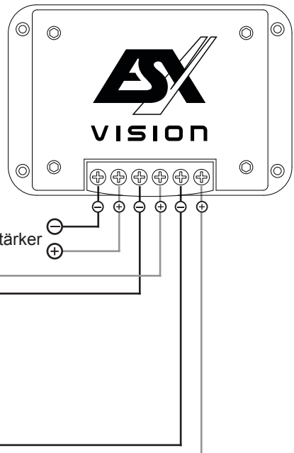
Frequenzweiche
