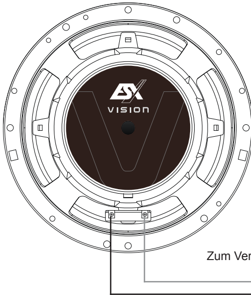
Tiefmitteltöner
