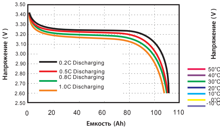
Графики разряда разными токами при 25°C
