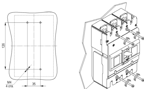
Рисунок 9 – Расположение отверстий для крепления выключателя на панели
