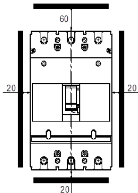
Рисунок 8 – Минимально-допустимые расстояния от выключателя до металлических частей
