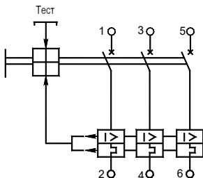
Рисунок 7 – Электрическая принципиальная схема выключателя
